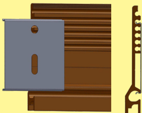
Clips di giunzione dei profili e aggancio meccanico alla muratura.
